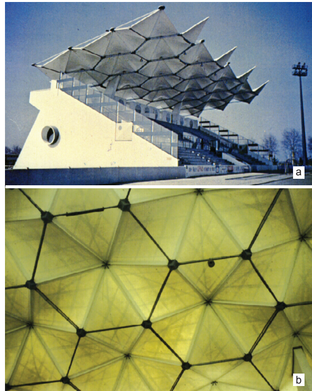
Il. 6. Laval Stadium: a) trybuny, b) detal pokrywy
