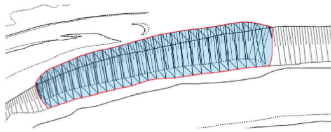
Fig. 6. Fragment of the triangulation surface of a mine block divided by parallel section planes Rys. 6. Fragment powierzchni triangulacyjnej bloku kopalnianego, podzielonego równoległymi płaszczyznami przekroju
