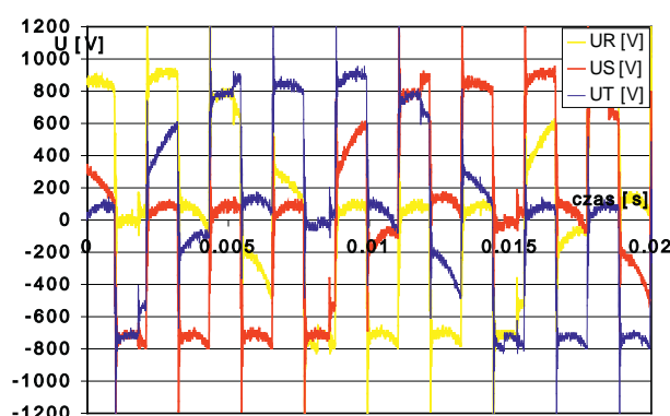
Rys. 2. Przebieg napięcia między fazami uzwojenia 590 V i kładź transformatora olejowego hermetycznego 670 kVA, 6/0,59 kV w czasie jednego okresu (20 ms)
