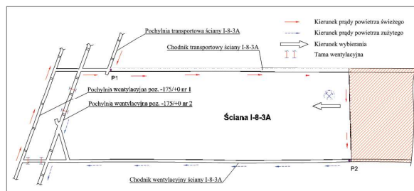
Rys. 2. Schemat przewietrzania rejonu ściany I-8-3A pokładu nr 8 w kopalni Vang Danh [15] Fig. 2. Diagram of the ventilation of the I-8-3A longwall area of the No. 8 seam at the Vang Danh mine [15]
