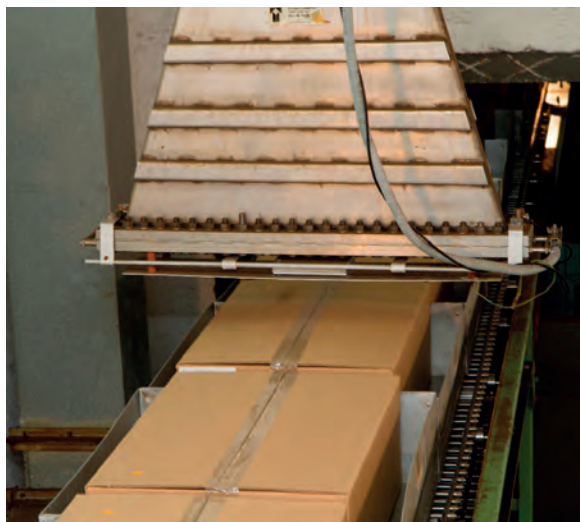
Ryc. 1 Radiacyjnie sterylizowane kartony ze sprzętem medycznym pod skanerem wiązki elektronów akceleratora Elektronika 10/10 w IChTJ
