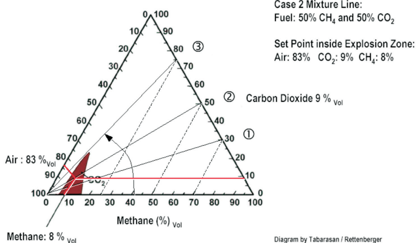
kys. 4. Tworzenie mieszanki: dodanie powietrza jako trzeciego składnika do \text{CO}_2 i \text{CH}_4
