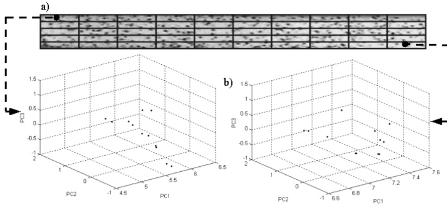
Rys. 2. Fragment klatki z mieszaniną dwóch materiałów sypkich, podzielony na obszary o tych samych rozmiarach ( L=50 ) (a); reprezentacja procesów elementarnych dwóch obszarów w trójwymiarowej przestrzeni głównych składowych (b)
