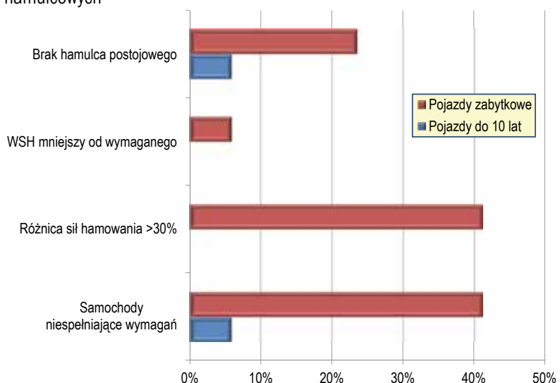
Rys. 2. Wyniki pomiarów przeprowadzonych na urządzeniu rolkowym i płytowym Źródło: oprac. własne.
