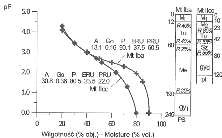
Rys. 1. Krzywe pF warstwy 10–20 cm oraz budowa stratygraficzna profilu gleby Mt Iba i Mt IIcc: popielność A (%), gęstość objętościowa Go ( \text{g}\cdot\text{cm}^{-3} ), porowatość P (% vol.), efektywna retencja użyteczna ERU (% vol.), potencjalna retencja użyteczna PRU (% vol.), M – mursz, Tu – torf turzycowiskowy, Sz – torf szuwarowy, Me – torf mechowiskowy, gy – gytia, pl – piasek luźny.
