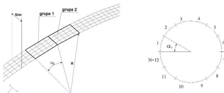
Rys. 10. Podział modelu MES linopędni na grupy obciążeń [opracowanie własne]
