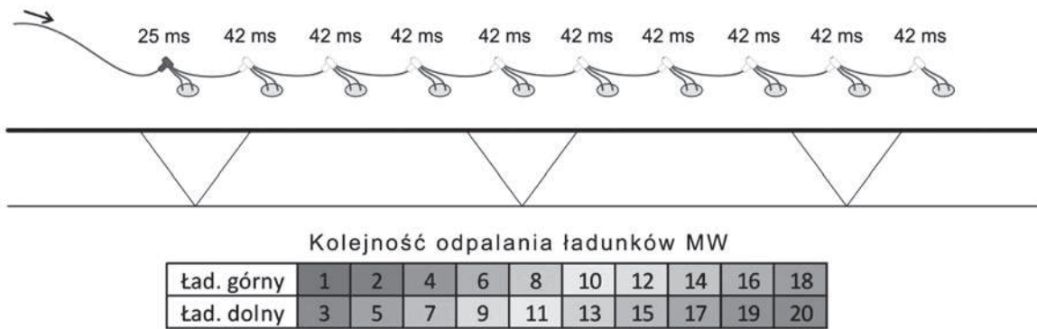
Rys. 1. Schemat połączenia nieelektrycznej sieci strzałowej w serii I wraz z kolejnością odpalanych ładunków MW Fig. 1. Blasting pattern with a charge firing sequence in the first series
