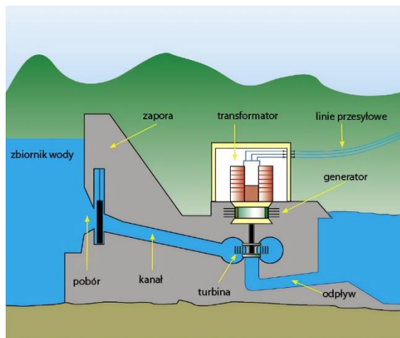
Rys. 2. Przekrój poglądowy elektrowni wodnej [8]
