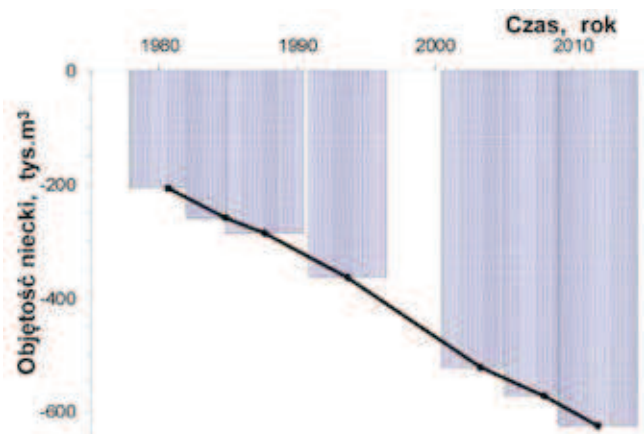
Rys. 3. Narastanie objętości niecki obniżeń powierzchni w Bochni w okresie 1978 ÷ 2011 r.
