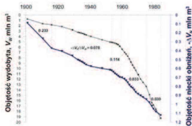
Rys. 5. Wydobycie i objętość niecki osiadań w Inowrocławiu [mln m³]
