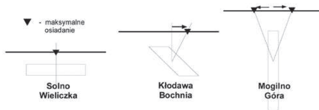
Rys. 14. Typy usytuowania się niecek osiadań; typ 1 – Solno, Wieliczka, typ 2 – Kłodawa, Bochnia, typ 3 – Mogilno, Góra
