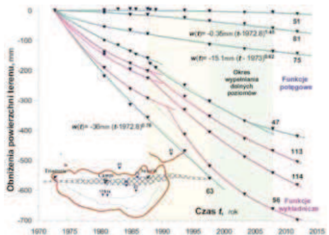
Rys. 7. Obniżenia reperów nad kopalnią w Bochni w okresie od 1972 do 2011 [mm]
