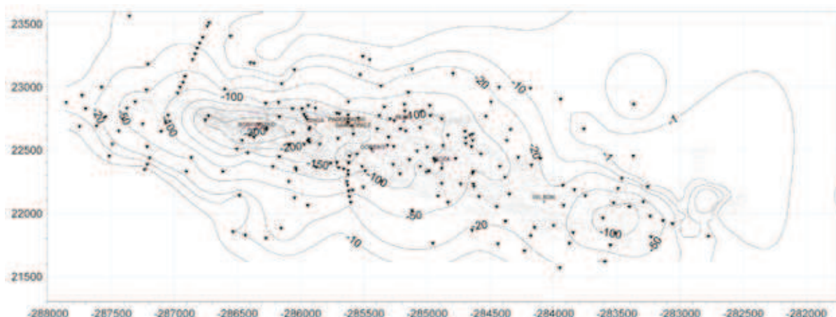
Rys. 9. Obniżenia terenu na kopalnię „Wieliczka” w okresie 1978 ÷ 1986 r. [mm] Fig. 9. Subsidence of terrain above the “Wieliczka” mine between 1978 and 1986 [mm]
