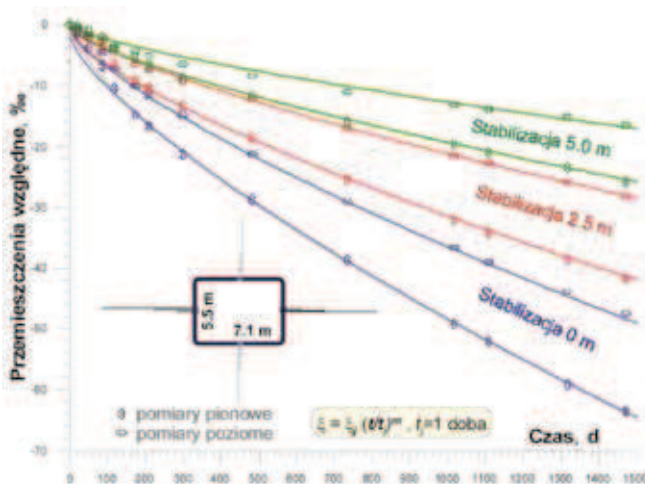
Rys. 2. Względne przemieszczenia i konwergencje chodnika w kopalni soli Sierszowice [31]; współczynniki funkcji (1) i długości baz pomiarowych: poziomych: m=0.725 ; \xi_j \in [0,245\%, 0,140\%, 0,085\%] , l \in [7,1 \text{ m}, 12,1 \text{ m}, 17,1 \text{ m}] pionowych: m=0.695 ; \xi_j \in [0,400\%, 0,260\%, 0,160\%] , l \in [5,5 \text{ m}, 10,5 \text{ m}, 15,5 \text{ m}]
