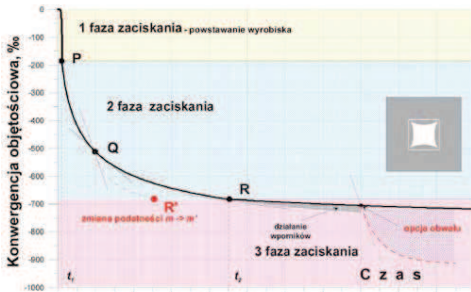
Rys. 1. Trzy fazy zaciskania wyrobiska
