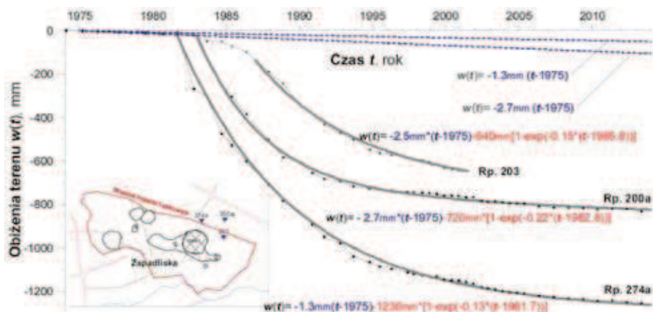
Rys. 8. Obniżenia reperów przy granicy złoża w Łęzkowicach w okresie 1974 ÷ 2001 [mm] Fig. 8. Subsidence of bench-marks at the deposit border in Łęzkowice between 1974 and 2001 [mm]
