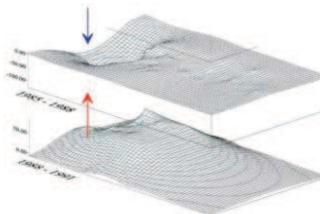
Rys. 25. Podnoszenie się 1 poziomu kopalni „Solno” w trakcie jej zatapiania [12]
