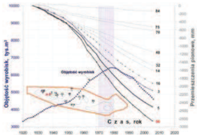
Rys. 6. Obniżenia reperów nad kopalnią w Wieliczce w latach 1926 ÷ 2006 [mm]
