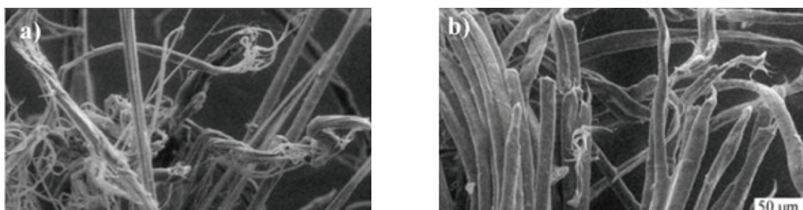
Rys. 5. Widok zniszczenia kompozytu wzmocnionego włóknem M5 (a) oraz Zylon® (b) podczas uderzenia pociskiem balistycznym [12]
