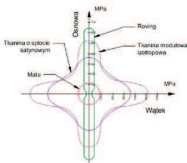
Rys. 4. Kierunkowa wytrzymałość laminatu z różnym wzmocnieniem szklanym [10]
