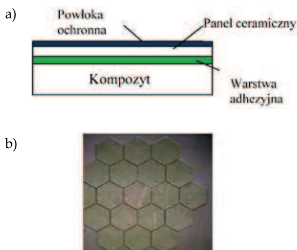
Rys. 2. Schemat (a) oraz widok panelu (b) lekkiej osłony balistycznej
