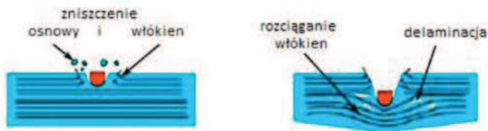
Rys. 3. Mechanizm dyssypacji energii uderzenia w procesie niszczenia kompozytu a) faza I – zniszczenie włókien i osnowy, b) faza II – delaminacja matrycy i rozciąganie włókien [7]
