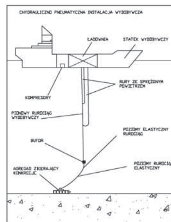
Rys 3. Hydrauliczno-pneumatyczna instalacja wydobywcza [1]
