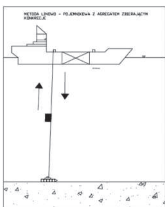
Rys 6. Metoda linowo-pojemnikowa z agregatem zbierającym конкреcje [1] Fig. 6. Rope-bin method with aggregate collecting concretions [1]
