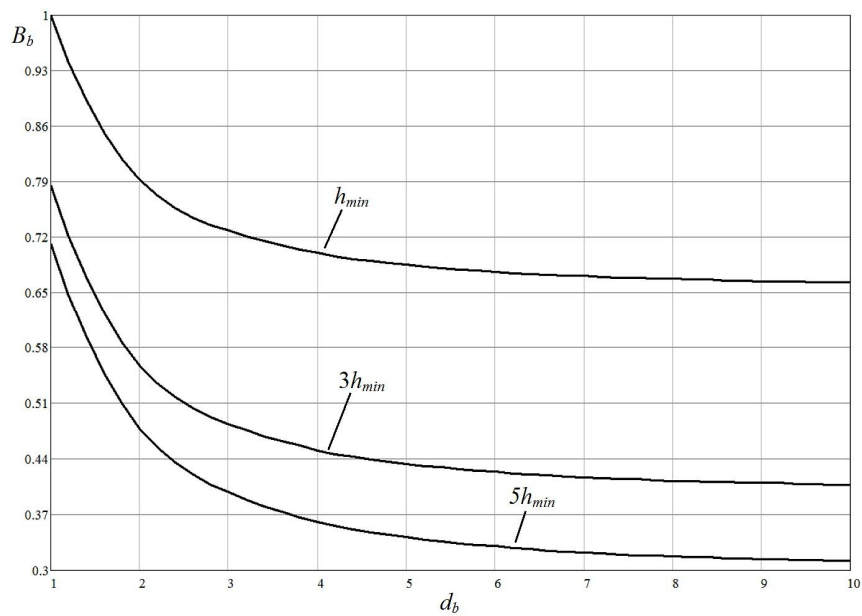
Rys. 4. Rozkład bezwymiarowej indukcji w funkcji bezwymiarowej odległości między przewodami d_b dla różnych odległości płyty od przewodu h = m \cdot h_{min}
