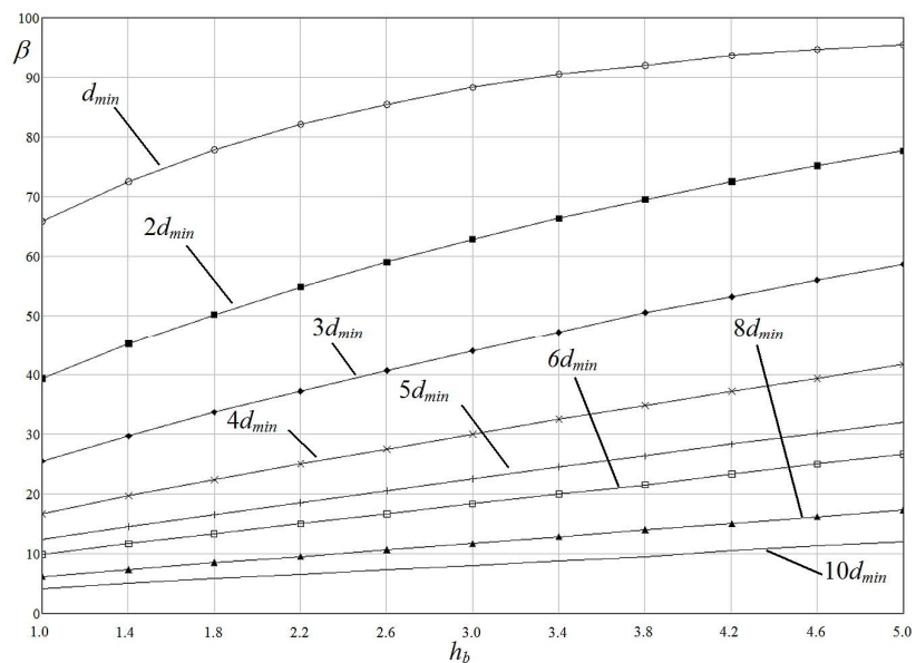
Rys. 3. Zależności bezwymiarowej wielkości \beta w funkcji bezwymiarowej odległości przewodu od płyty h_b dla różnych odległości pomiędzy przewodami d = k \cdot d_{min}
