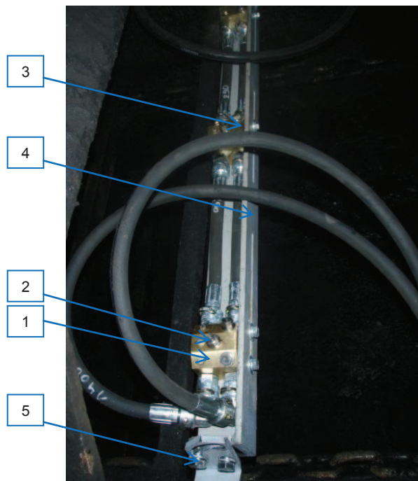
Rys. 4. Bateria zraszająca systemu PASAT [7]
