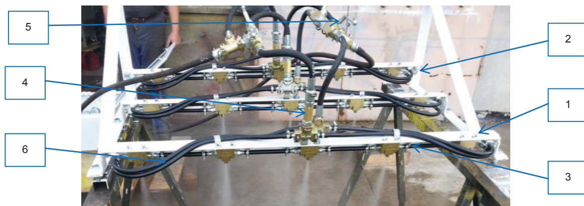
Rys. 11. Zespół zraszający podczas prób ruchowych u producenta [7]
