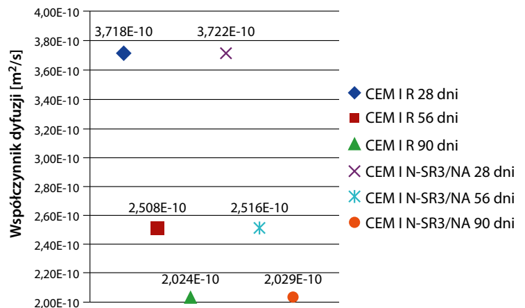
Wykres 5. Wartości współczynników dyfuzji w stanie nieustalonym w zależności od cementu i wieku próbki [19]
