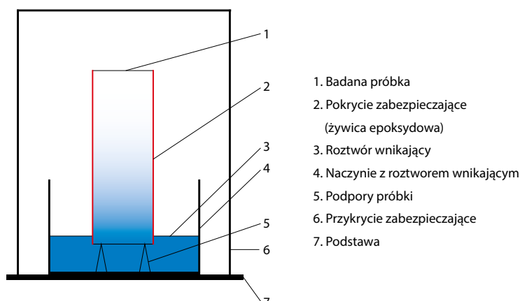
Rysunek 1. Schemat badania dyfuzji chlorków w stanie nieustalonym
