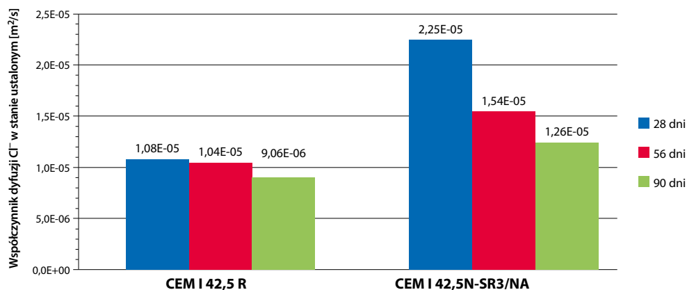
Wykres 7. Porównanie współczynników dyfuzji w stanie ustalonym w zależności od rodzaju cementu i wieku próbki [18]
