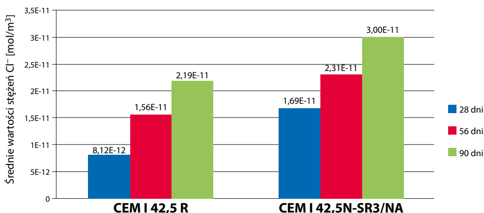
Wykres 6. Wyniki zawartości chlorków w stanie ustalonym w zależności od rodzaju cementu i wieku próbki [19]
