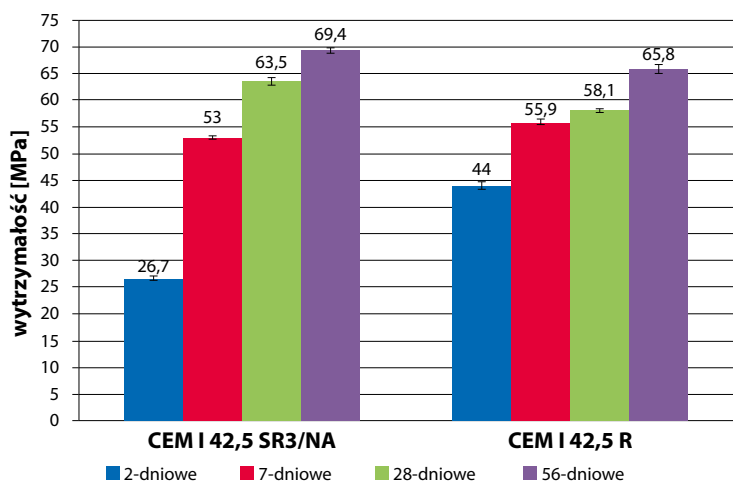
Wykres 2. Średnie wytrzymałości na ściskanie badanych betonów [18]
