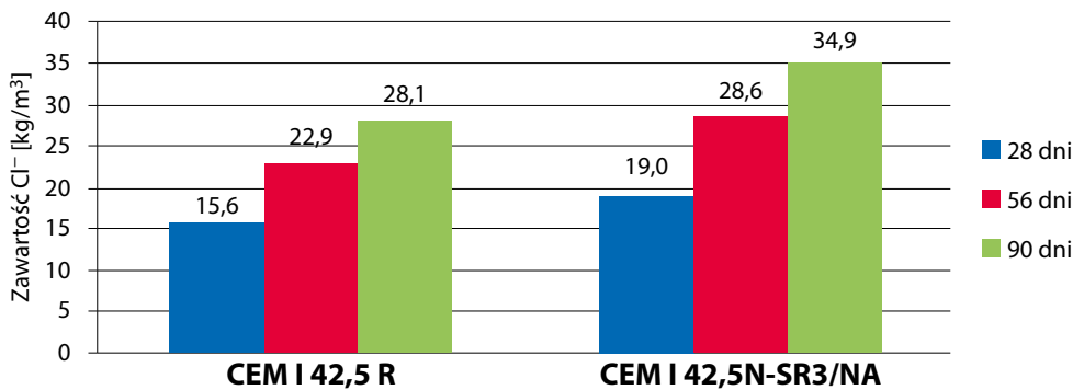
Wykres 4. Zawartość jonów chlorkowych w próbkach zapraw w zależności od czasu oddziaływania stężonego NaCl [19]
