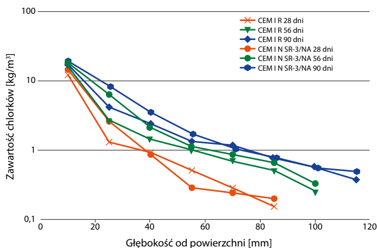
Wykres 3. Wyniki zawartości chlorków w stanie nieustalonym w czasie od 28 do 90 dni oddziaływania nasyconego NaCl w zależności od głębokości warstwy [19]
