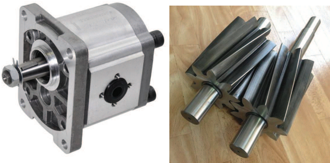
Rys. 4. Pompa zębata o uzębieniu skośnym [7, 8]
