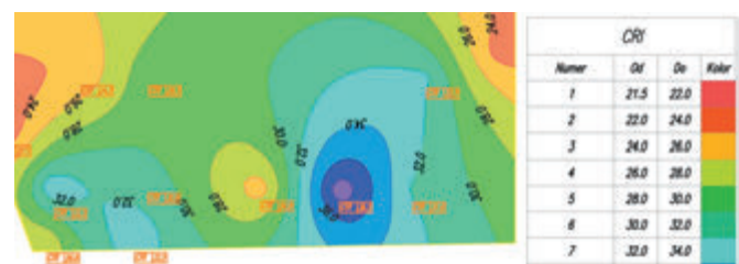
Rys. 1. Mapa właściwości koksotwórczych węgla Fig. 1. The map of coking properties of coal
