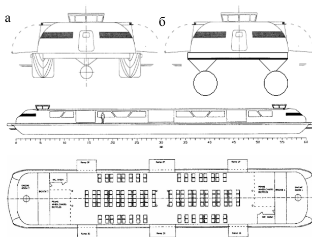
Рис. 7. Многокорпусный речной трамвай; вид спереди, вид сбоку, вид на пассажирскую палубу [11]
