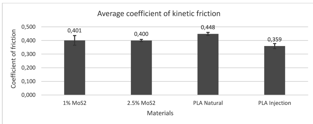
Fig. 10. Comparison of kinetic friction coefficient values for all materials Rys. 10. Zestawienie porównawcze wartości współczynnika tarcia kinetycznego wszystkich materiałów
