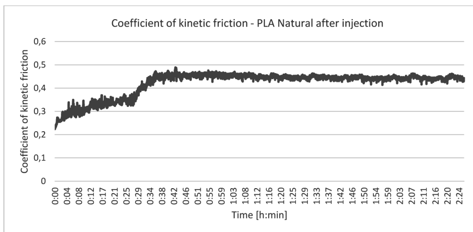
Fig. 8. Values of the kinetic friction coefficient during the whole test – PLA Natural after injection process Rys. 8. Wartości współczynnika tarcia kinetycznego w trakcie całego badania – PLA Natural po procesie wtrysku
