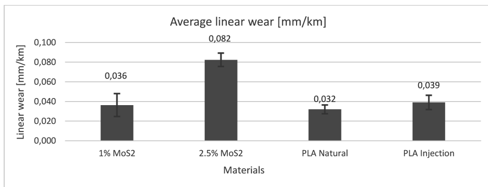
Fig. 9. Comparison of linear wear values for all materials Rys. 9. Zestawienie porównawcze wartości zużycia liniowego wszystkich materiałów
