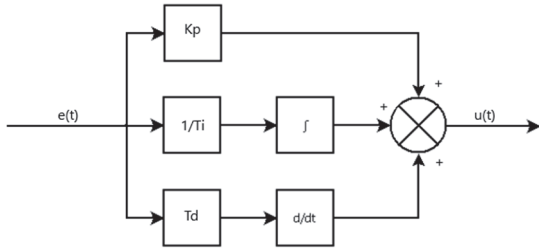
Rys. 7. Schemat blokowy regulatora PID Fig. 7. Block scheme of PID controller
