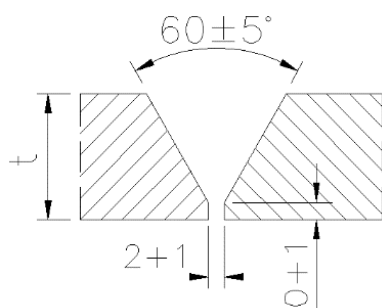
Rysunek 1 Sposób ukosowania złącza trójsięgowego
