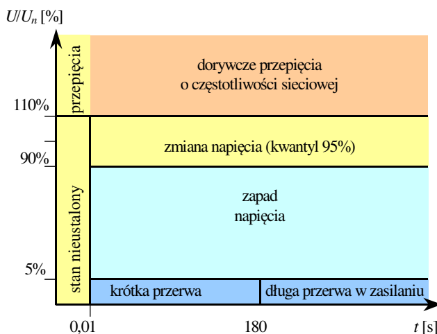
Rys. 1. Klasyfikacja zaburzeń ze względu na wartość skuteczną napięcia U_{rms} i czas trwania zaburzenia t
