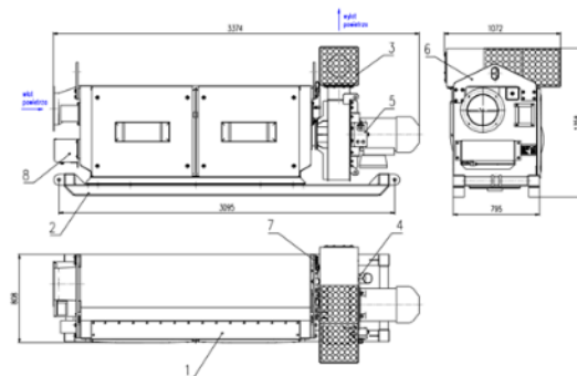
Rys. 4. Budowa prototypowego odpylacza suchego: 1 – zespół oczyszczania powietrza, 2 – zespół odbioru zanieczyszczeń, 3 – dyfuzor, 4 – uchwyt złącza kablowego, 5 – pulpit sterowniczy, 6 – zawieszanie, 7 – zespół pneumatyczny, 8 – pneumatyczne sterowanie czyszczeniem [2]
