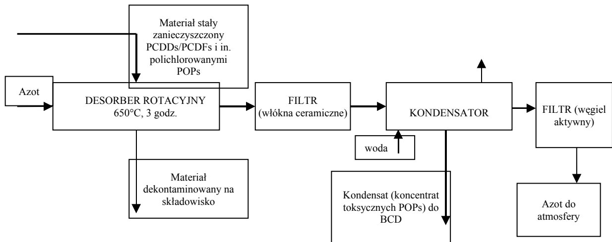
Rys. 1. Uproszczony schemat technologii pośredniej desorpcji cieplnej (ITD) dioksyn (PCDDs/PCDFs) i innych polichlorowanych POPs ( Persistent Organic Pollutants ) z materiałów stałych o małym stężeniu kontaminantów
