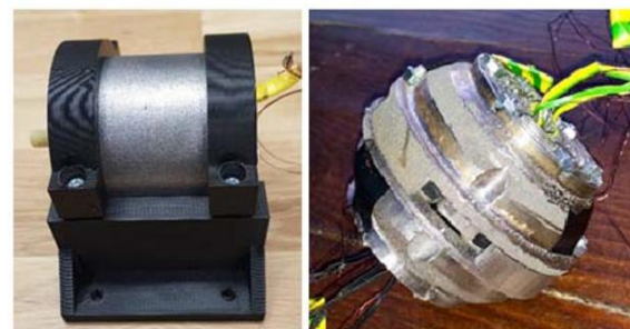
Rys. 5. Silnik reluktancyjny z a) promieniowym b) osiowym rozkładem pola [10]
