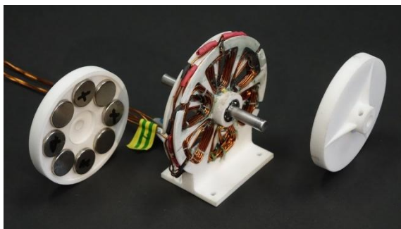
Rys. 8. Silnik tarczowy [15]
