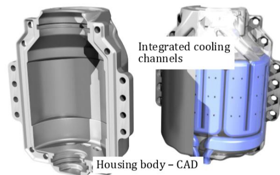
Rys. 10. Obudowa silnika elektrycznego ze zintegrowanymi kanałami do chłodzenia cieczą, a) model CAD oraz wykonana obudowa – Technical University of Munich, b) model CAD – University of Nottingham[6],[7]
