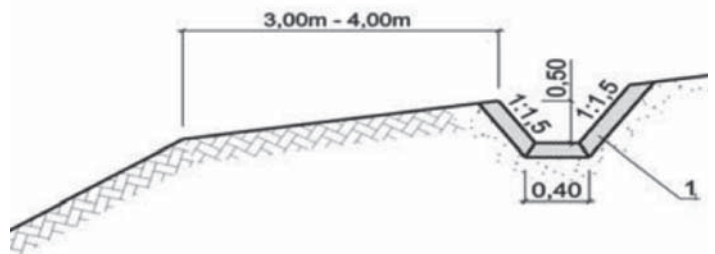
Rys. 7. Przykład umocnienia rowu stokowego geosyntetykami
