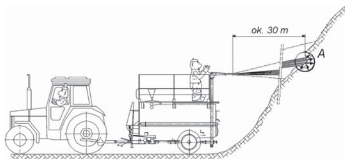
Rys. 13. Hydrodynamiczne nanoszenie komponentu siewnego formującego warstwę ochronną na skarpie
