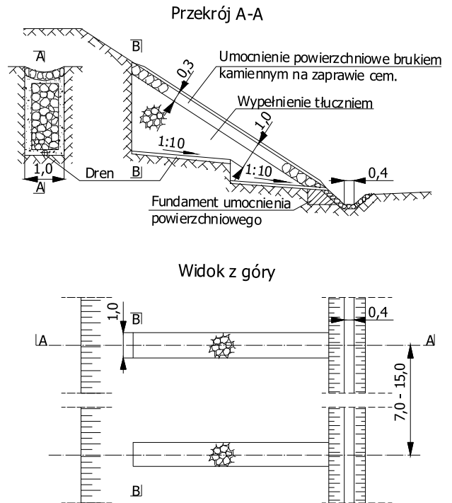
Rys. 9. Drenowanie wgłębne poprzeczne odwadniające
