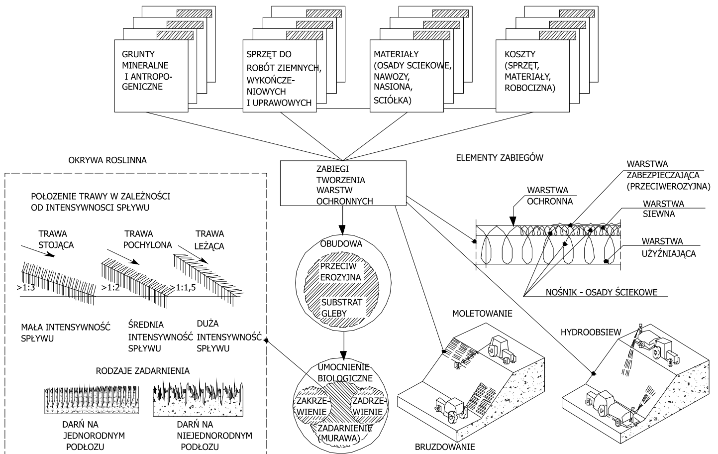
Rys. 12. Schemat zabiegów agrogeotechnicznych przygotowujących skarpy do zadarnienia metodą hydroobsiewu
