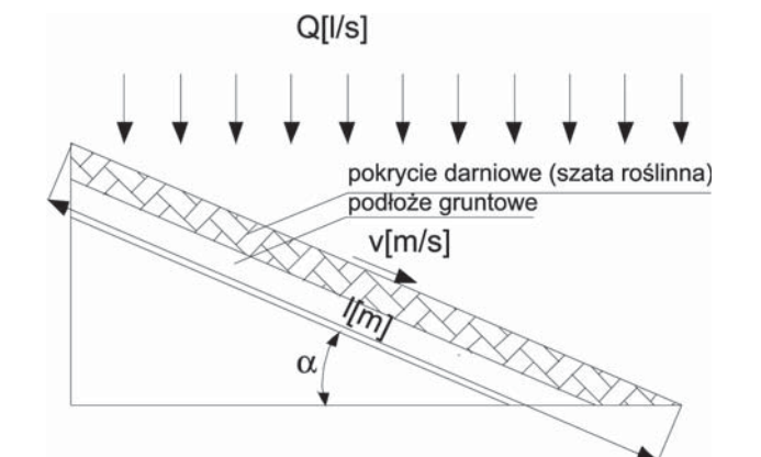
Rys. 2. Schemat intensyfikacji erozji zależnie od opadu i kąta nachylenia skarpy
