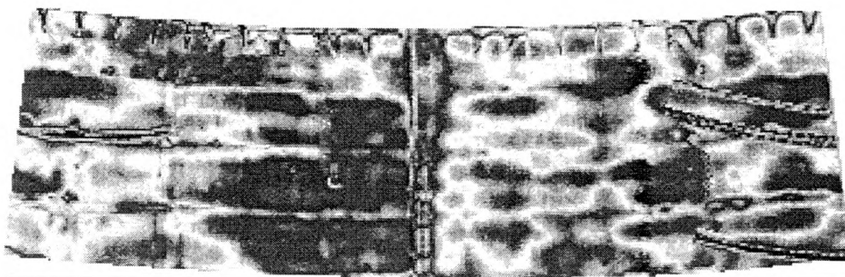
Rys. 6. Mozaika rozwinięć obrazów termograficznych fragmentu kominia
