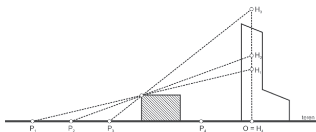
Il. 1. Ogólny schemat metody VIS – relacja punktów obserwacji ( P ) i progów widoczności badanego obiektu ( H ) (oprac. K. Czyńska, P. Rubinowicz)
