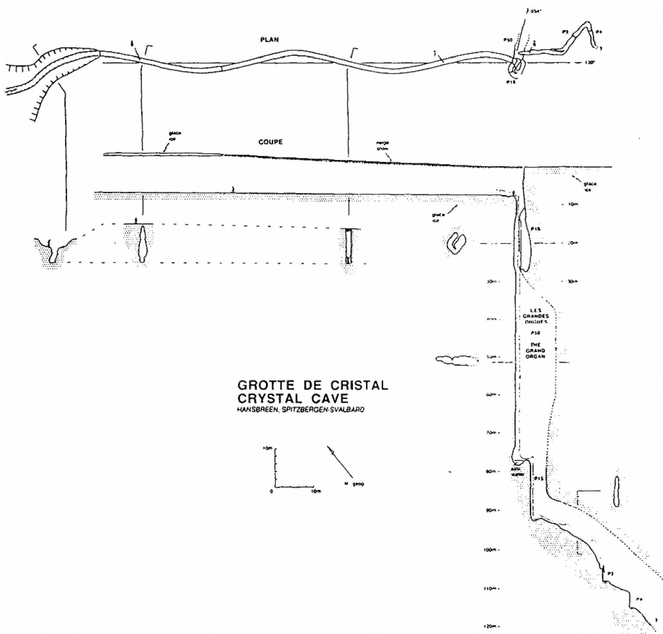
Fig. 15. Grotte de Cristal in Hansbreen (Schroeder 1995)
