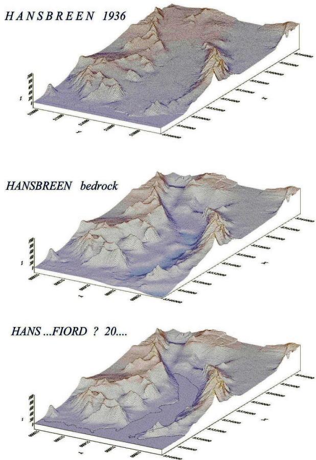
Fig. 26. DTM models of Hansbreen (Kolondra 1993)
