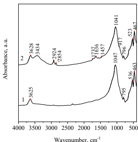
Fig. 3. IR spectra of: 1) MMT, 2) MMT- co -MA/AA
