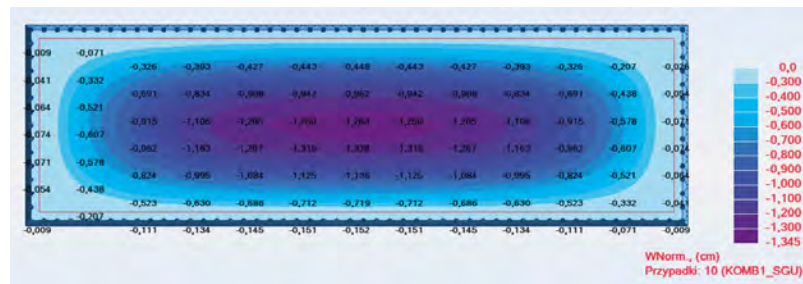
Rys. 5. Ugięcia – szyba GL 2 1430 x 4900 (66.2); ciężar własny (wsp. bez. 1,0), siła pozioma (wsp. bez. 0,2), parcie wiatru (wsp. bez. 0,9), ssanie wewnętrzne (wsp. bez. 0,2), ciśnienie izochoryczne (wsp. bez. 0,2), źródło: archiwum własne autora – dokumentacja projektowa
