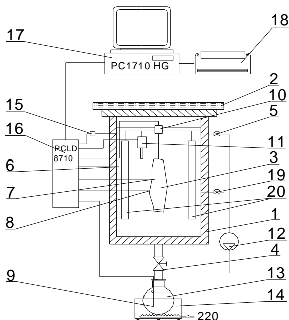
Rys. 2. Schemat stanowiska badawczego:
