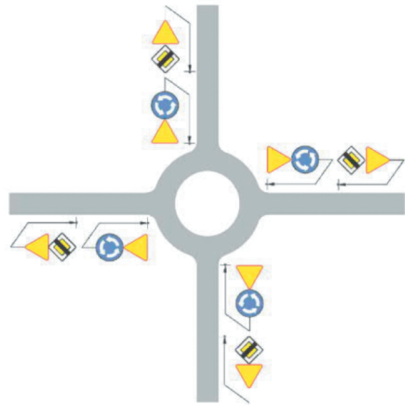
Rys. 1. Schemat skrzyżowania w ruchu okrężnym
