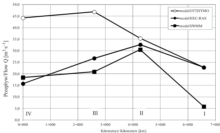
RYSUNEK 3. Przepływy maksymalne o prawdopodobieństwie przekroczenia 1% obliczone przy zastosowaniu różnych modeli w czterech przekrojach obliczeniowych FIGURE 3. Maximum flows with probability of exceedance of 1% calculated using different models in four cross-sections
