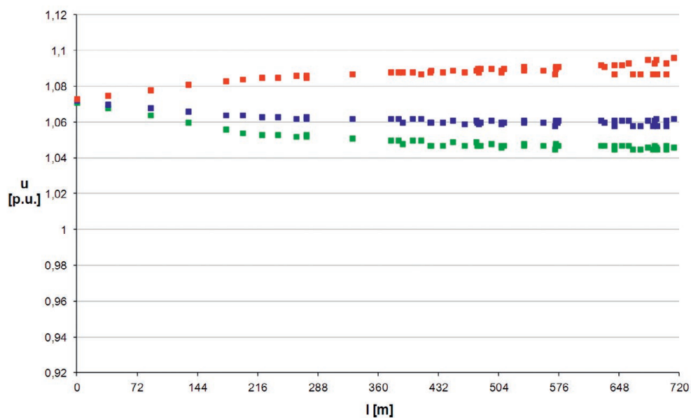
Rys. 5. Poziomy napięć przy minimalnym obciążeniu systemu: ■ brak generacji, ■ praca elektrowni wiatrowych z mocą równą 30% mocy znamionowej, ■ praca elektrowni wiatrowych z mocą znamionową
