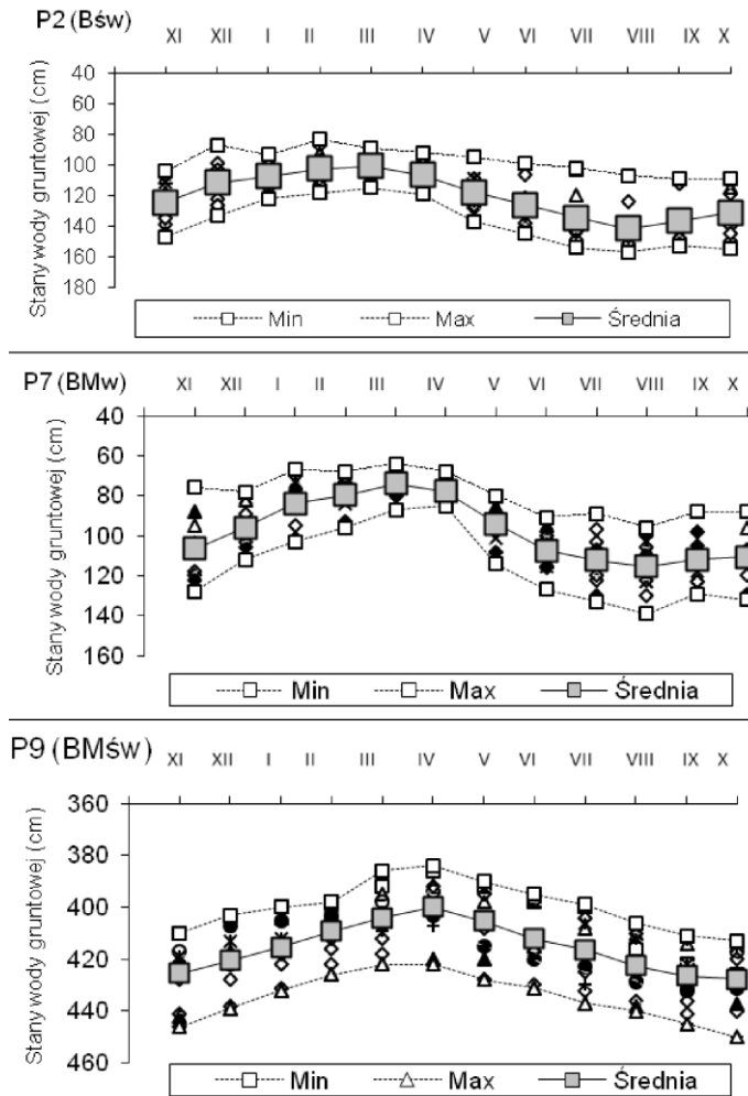
Rys. 3. Przebieg średnich, min i max miesięcznych, stanów wody gruntowej w badanych siedliskach zlewni cieku Potaszka w latach 1998–2007
