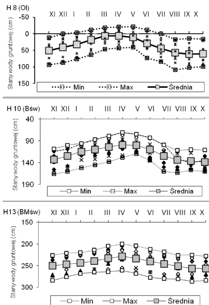
Rys. 2. Przebieg średnich, min i max miesięcznych, stanów wody gruntowej w badanych siedliskach zlewni ciek Hutka w latach 1998–2007
