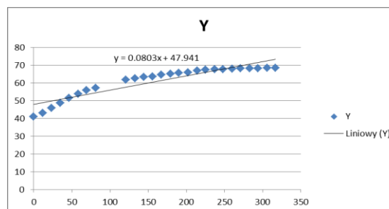
Rys. 22 Zmiana obrotów w zakresie 100-120 obr/min, docisk ośki do powierzchni gładzonej p=0,5 MPa
