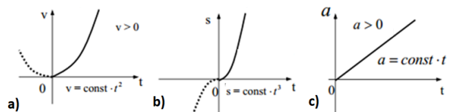
Rys. 5 Trajektorja ruchu ziarna „VH” w ruchu niejednostajnie przyspieszonym: a) prędkość ziarna, b) droga, c) przyspieszenie
