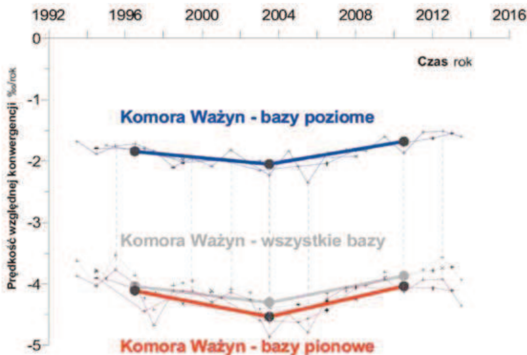
Rys. 15. Prędkości konwergencji względnej poziomej i pionowej w komorze Wążyn (opracowanie własne)
