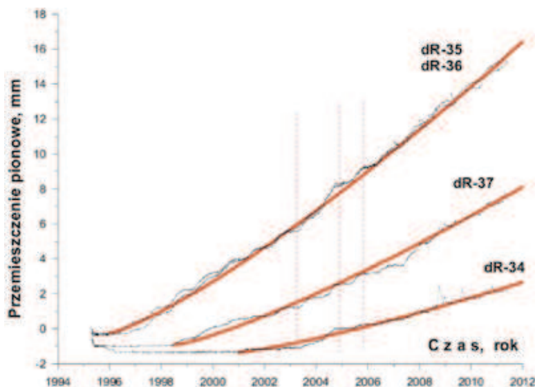
Rys. 8. Przemieszczenia stropu mierzone czujnikami ruchu dR w komorze Warszawa [14]
