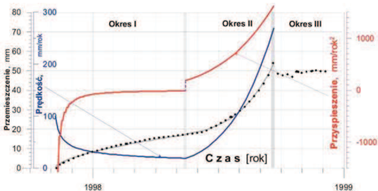
Rys. 11. Przemieszczenia, ich prędkości i przyspieszenia zarejestrowane w komorze Gołuchowski przed obwalem stropu [11]
