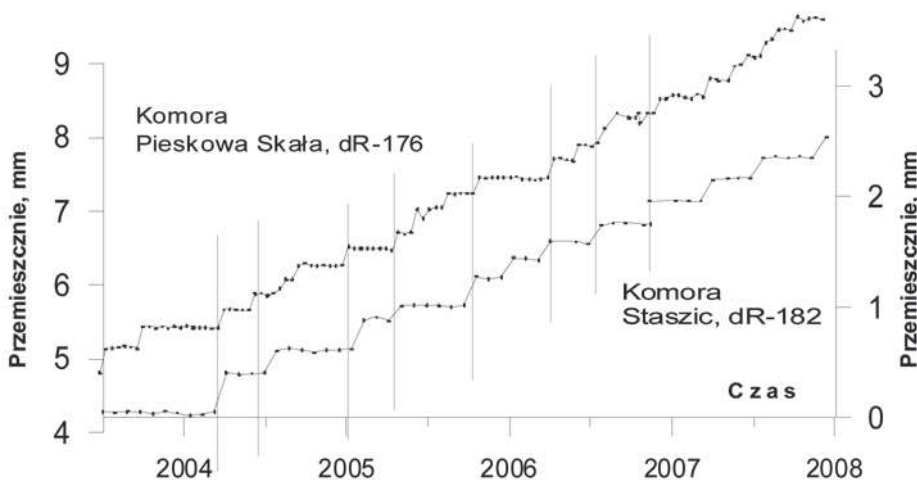
Rys. 9. Koordynacja ruchu periodycznego w stropie komór Pieskowa Skala i Staszic w kopalni Wieliczka [14]
