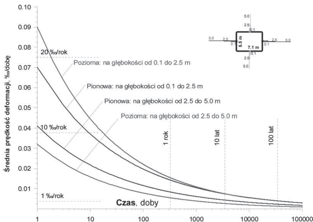
Rys. 13. Deformacje liniowe calizn w otoczeniu chodnika w kopalni soli Sieroszowice (opracowanie własne)
