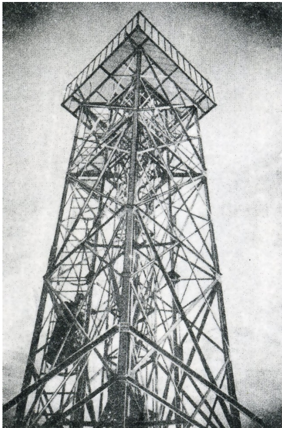
Rys. 4. Maszt nadawczy na dachu budynku Prudential
