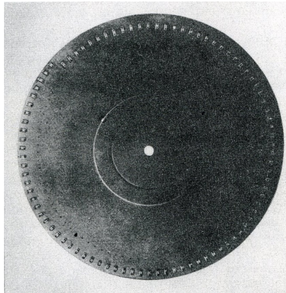
Rys. 1. Tarcza Nipkowa dla systemu telewizji 90-liniowej wykonana w 1936 r. w Państwowym Instytucie Telekomunikacyjnym w Warszawie
