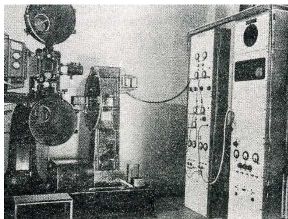
Rys. 3. Aparat telekinematograficzny na bazie projektora typu Ernemann V
