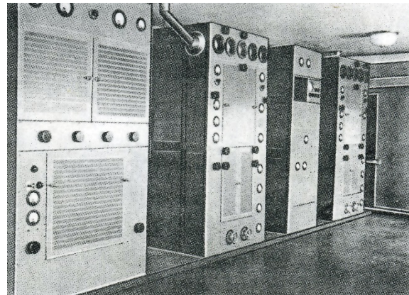
Rys. 5. Nadajniki obrazu i dźwięku zainstalowane na poddaszu Prudentialu
