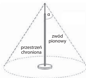
Rys. 4. Strefa ochronna zwodu Franklina
