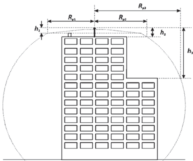
Rys. 5. Strefa zwodu ESE umieszczonego na dachu budynku wg normy NF C 17102. Długość strefy ochrony oznaczona jako R_p jest znacznie większa niż klasycznego zwodu Franklina umieszczonego w tym samym miejscu i o tej samej wysokości
