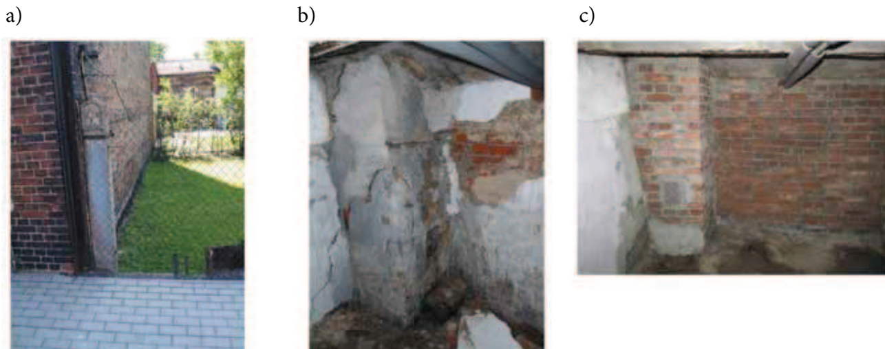
Rys. 2. Budynek lp.1: a) widok ściany szczytowej – wpełnięcie do piwnic budynku, b) uszkodzenie wewnątrz budynku, c) po remoncie
