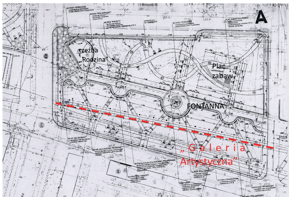
Ryc. 2. Plan zagospodarowania Placu Grunwaldzkiego w Katowicach z „Galerią Artystyczną”. (projekt „Pracownia Projektowa A. i A. Grzybowski – Architekci”, 2002 r.).
