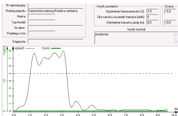
Rys. 3. Sprawny układ hamulcowy. Maksymalne opóźnienie hamowania 7,9 m/s 2 , czas hamowania 2,9 s
