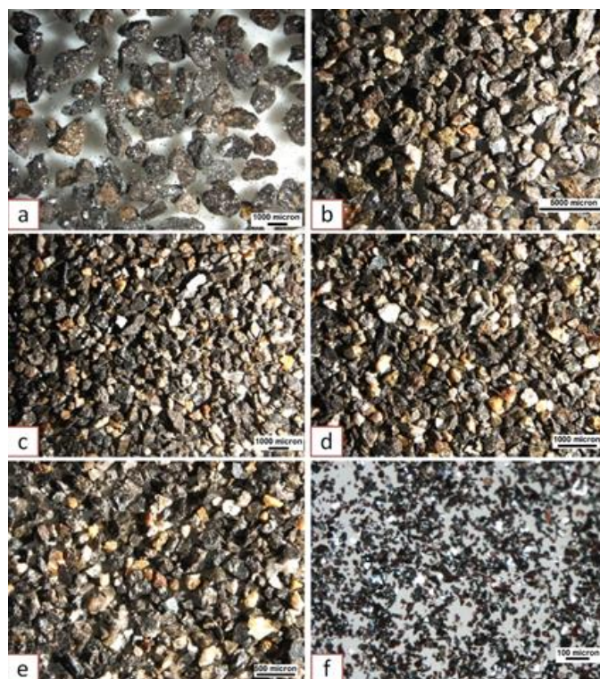
Fig. 2. Pictures of different size fractions (a) 2-1 mm (b) 1000-600 \mu\text{m} (c) 600-400 \mu\text{m} (d) 0.4-0.212 mm € 212-106 \mu\text{m} (f) -106 \mu\text{m}
