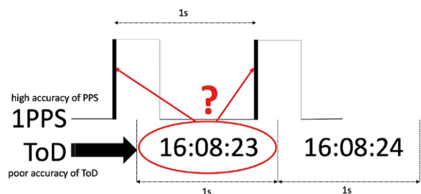
Rys. 21. Który z sygnałów 1PPS (lewy czy prawy) prawidłowo określa początek znacznika ToD godziny 16:08:23
