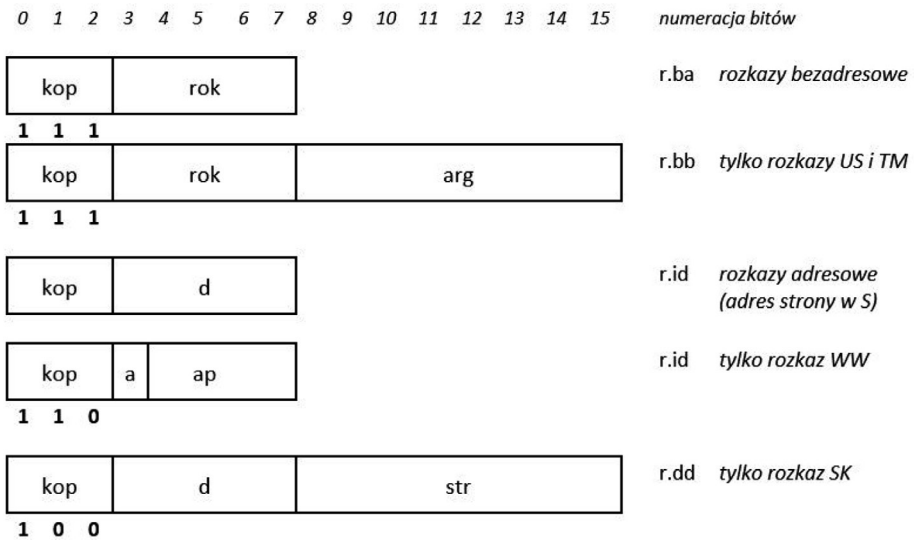
Rys. 1. Formaty rozkazów procesora Momik 8b
