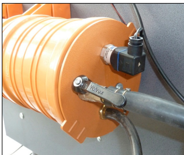
Rysunek 2. Układ stabilizacji podciśnienia Figure 2. The under pressure stabilization system
